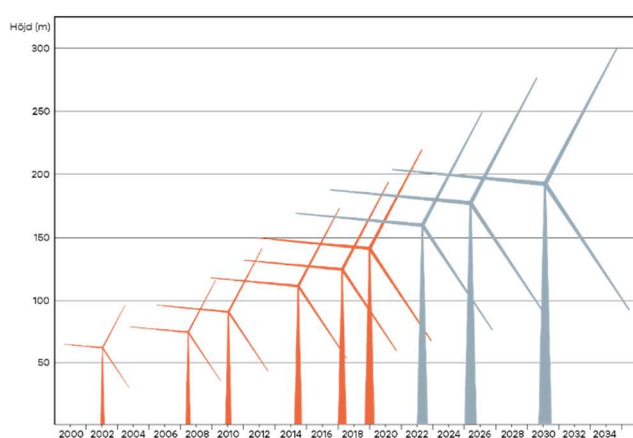
Figur 8. Vindkraftverken blir större och mer effektiv.
