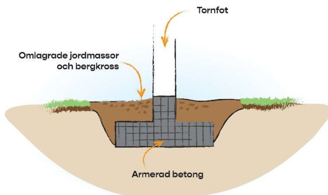
Figur 9. Illustration på Gravitationsförankrat fundament.
