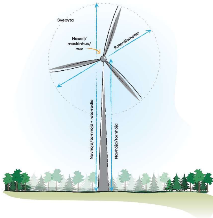
Figur 7. Vindkraftverk och definitioner.
