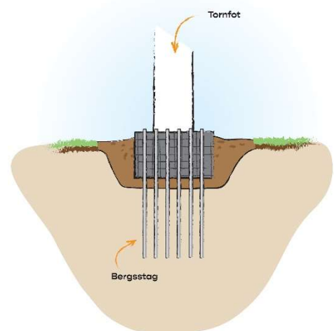
Figur 10. Illustration på Bergsförankrat fundament.
